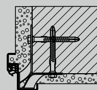
Монтаж при помощи дюбельных анкеров
