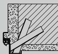
Монтаж при помощи анкеров для кирпичной кладки
