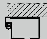
Блочная коробка для монтажа на стене (профиль 006) (испытано на стороне, противоположной стороне петель)
