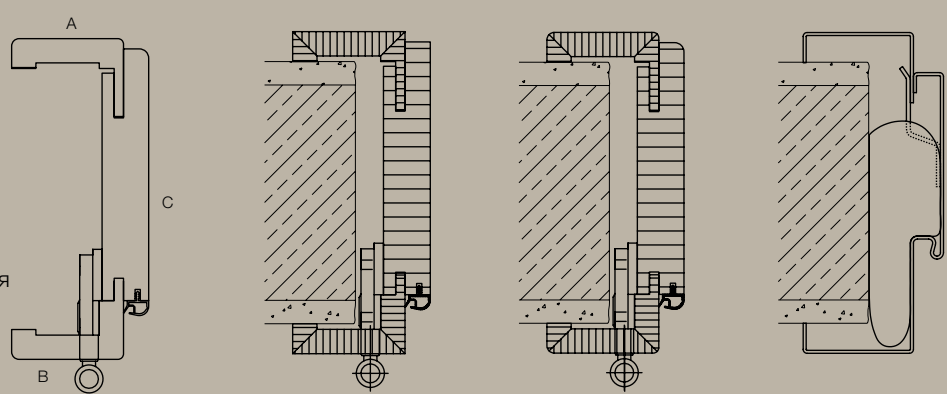
А: декоративная облицовка В: облицовка фальца С: добор коробки Деревянная коробка, прямоугольные кромки Деревянная коробка, закругленная кромка Стальная облицовочная коробка VarioFix
